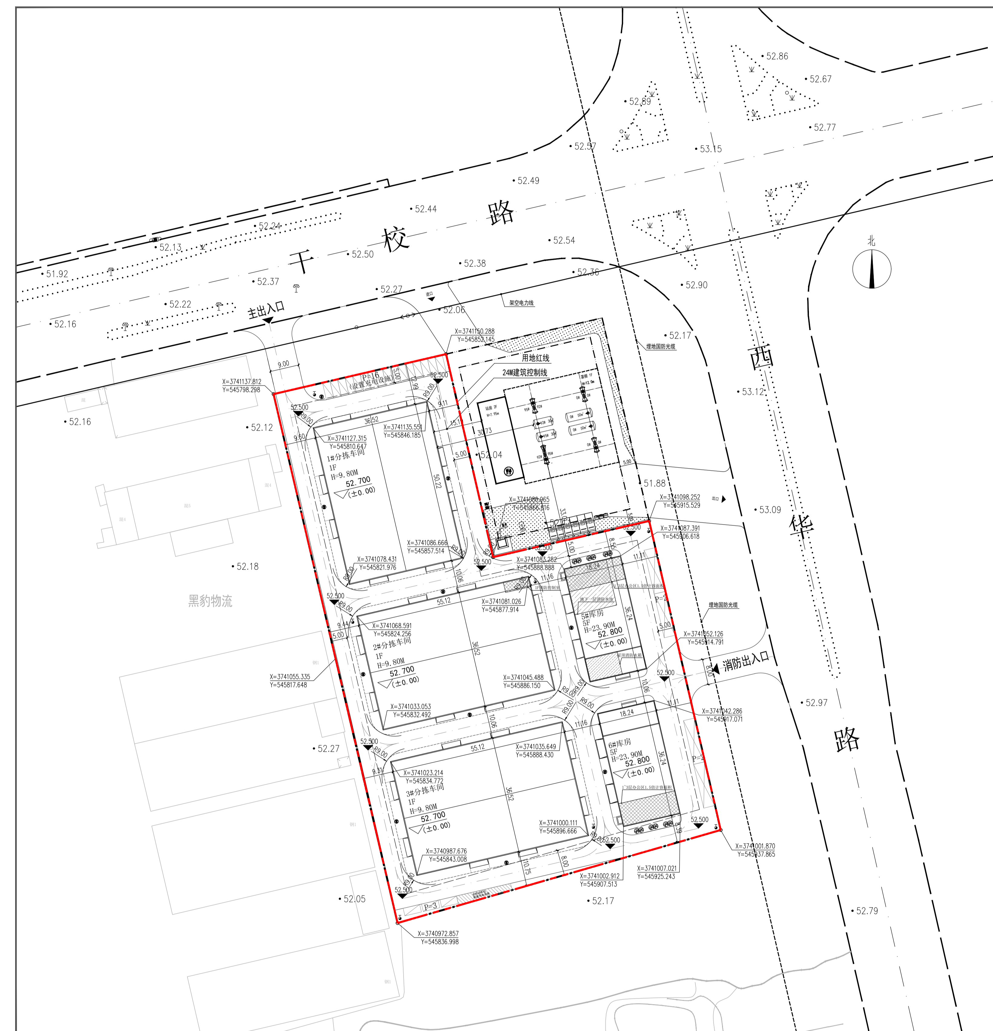
总平面布置图
