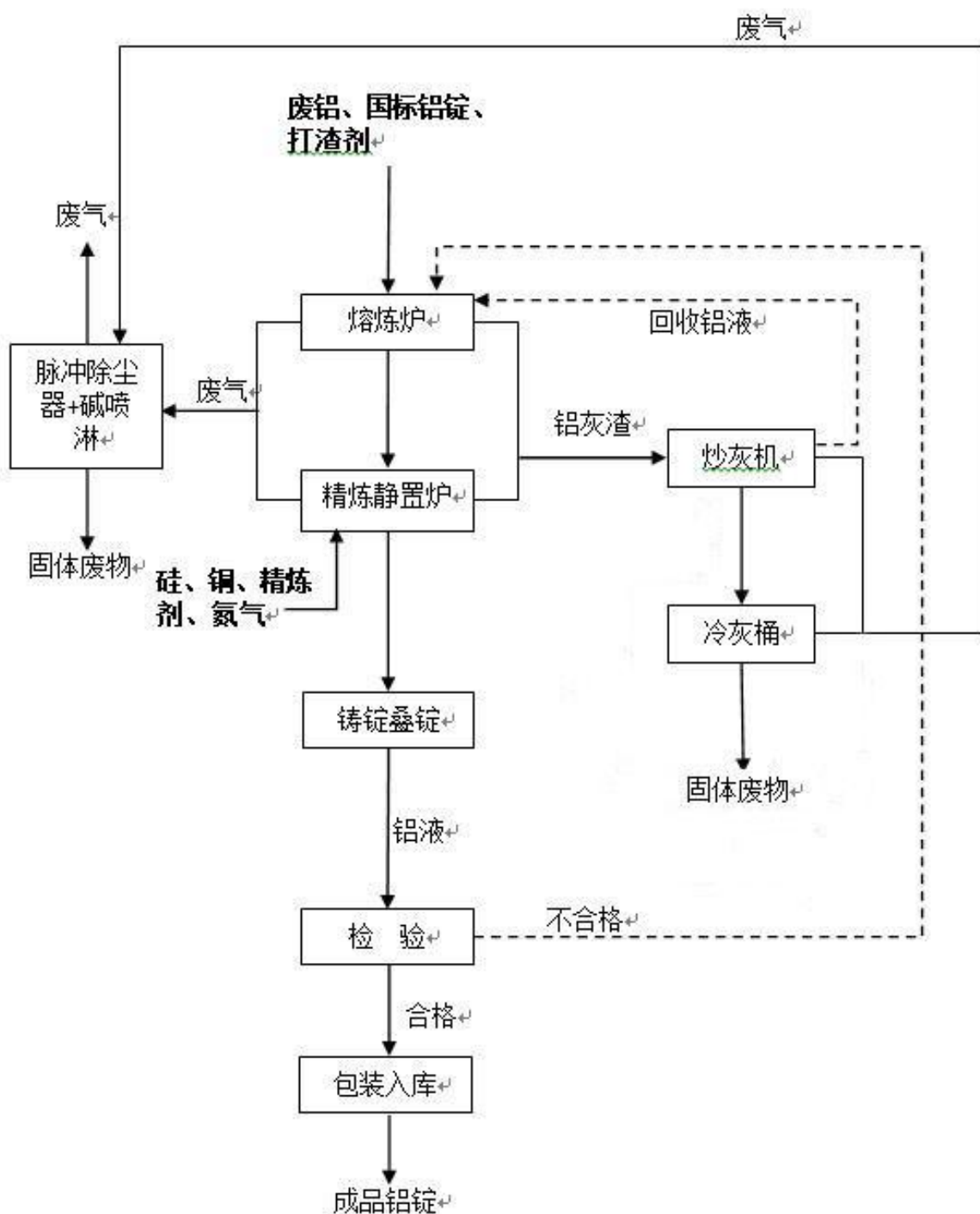
图4-1 生产工艺流程图及产污环节示意图
