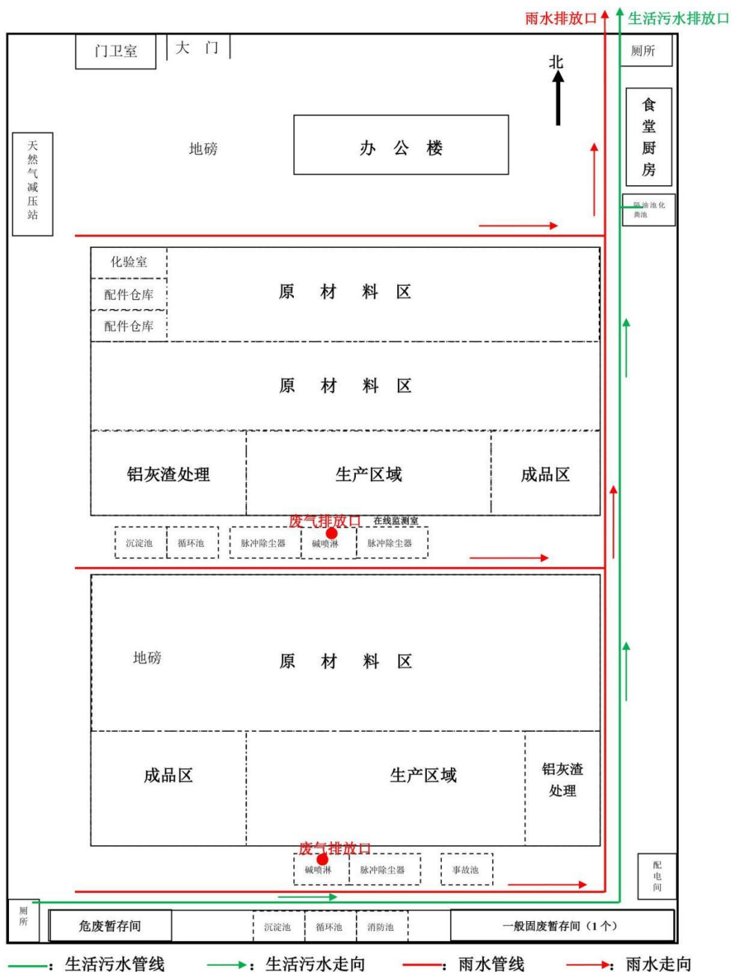
图4-2 平面布置图
